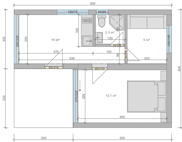
MODULHAUS KING-CAB Gesamfläche - 39 m 2 Wohnfläche - 30.4 m 2
