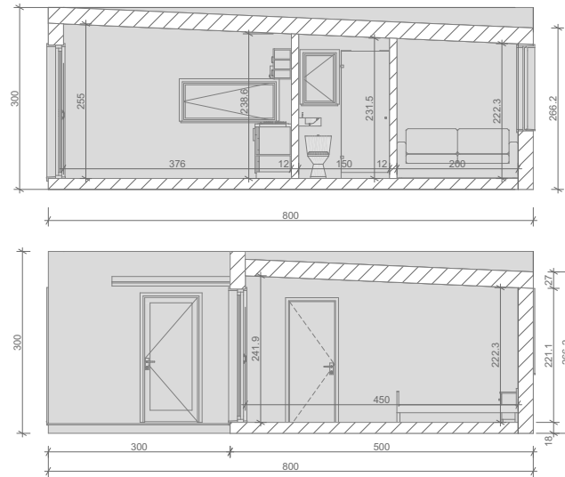
MODULHAUS KING-CAB Gesamfläche - 39 m 2 Wohnfläche - 30.4 m 2
