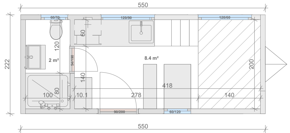
TINY NOMAD Gesamtfläche - 12.3 m 2 Wohnfläche - 10.4 m 2
